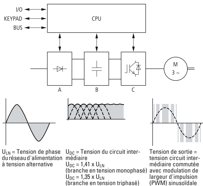
Schéma fonctionnel avec principaux composants d'un convertisseur de fréquence
